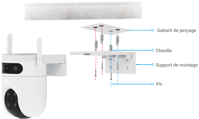
Fig. 1 Montage au plafond
